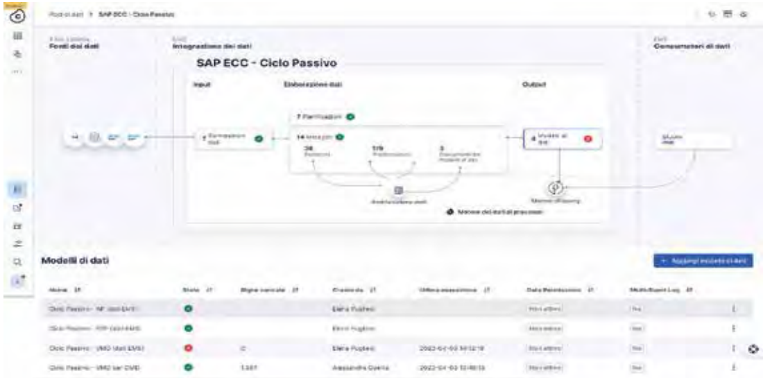
Figura 3: Schermata Celonis del Data Model
